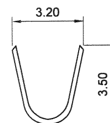
A-A SECTION
